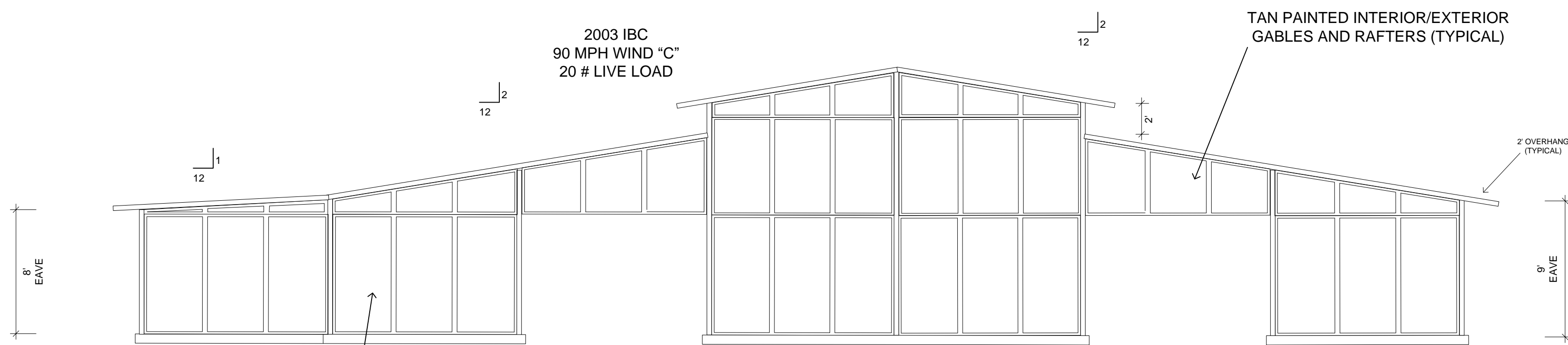
END ELEVATION
